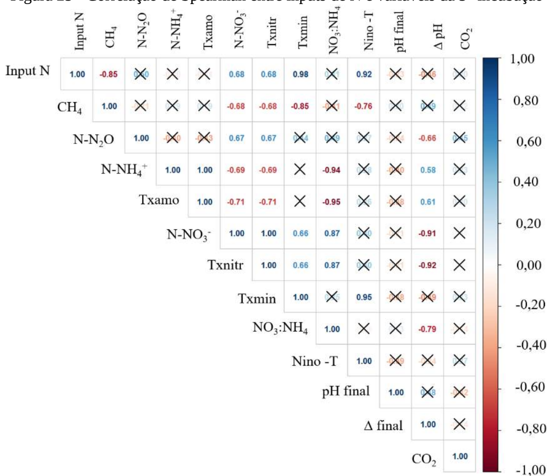
Figura 25 - Correlação de Spearman entre inputs de N e variáveis da 3ª incubação
