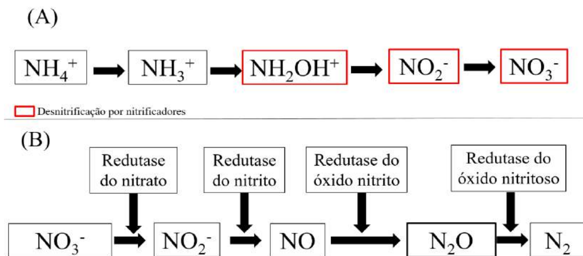
Figura 4 – Processos de Nitrificação (A) e Desnitrificação (B), envolvidos na produção de N 2 O
