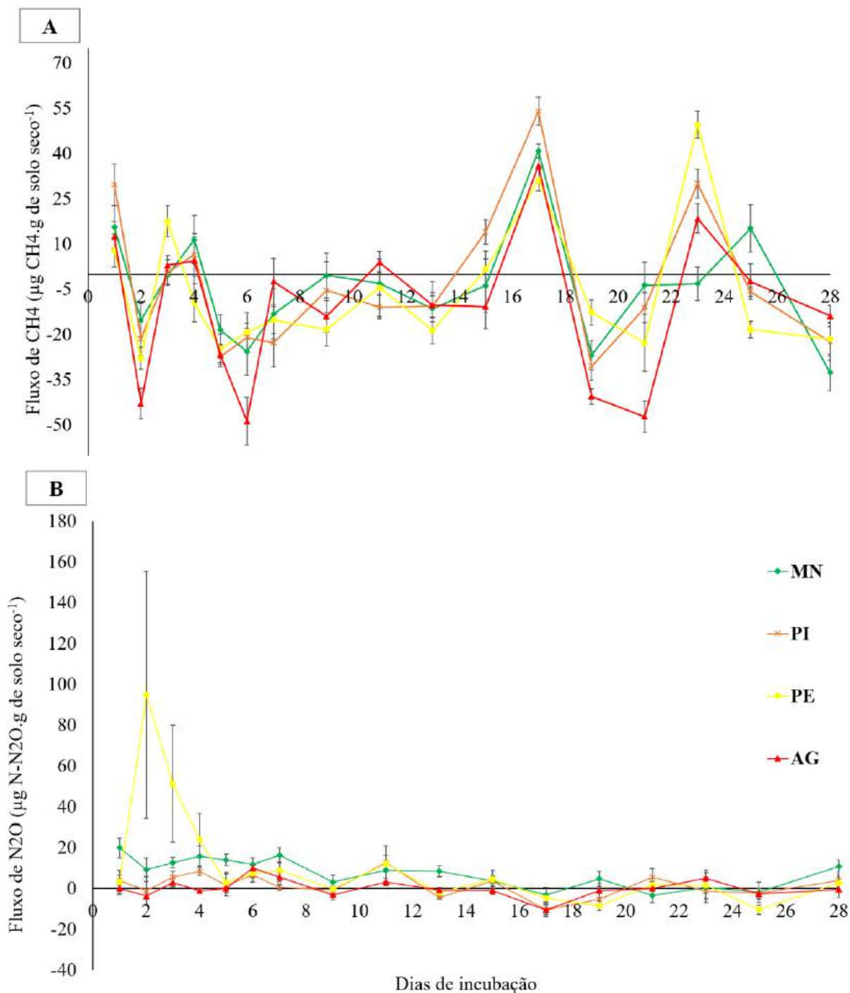
Figura 10 - Fluxo de metano ( \text{CH}_4 ) (A) e óxido nitroso ( \text{N}-\text{N}_2\text{O} ) em função do uso da terra ( 1^\circ incubação)
