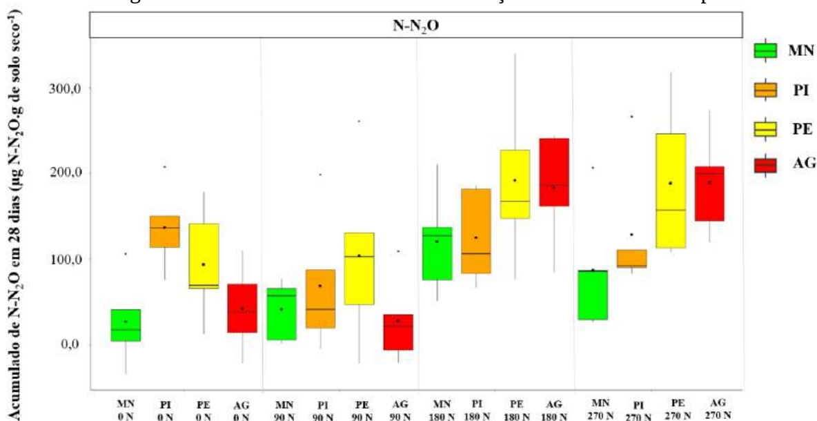
Figura 21 - Acumulativo de N-N 2 O em função do uso da terra e inputs de N
