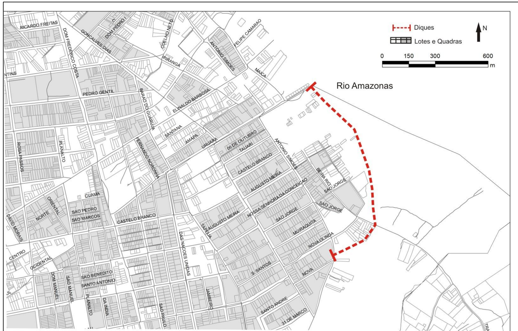
Figura 23 - Estrutura do dique de contenção que margeia no bairro Uruará.
