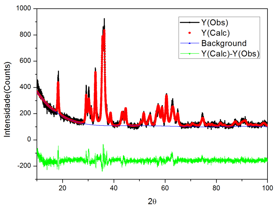
Figura 17 – Difratoograma experimental (preto), calculado (vermelho), a diferença entre o calculado e o observado (verde) e o background (azul), para a amostra N25CM900.
