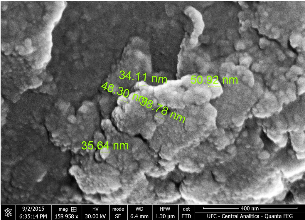
Figura 26 – Micrografia da amostra NM900.
