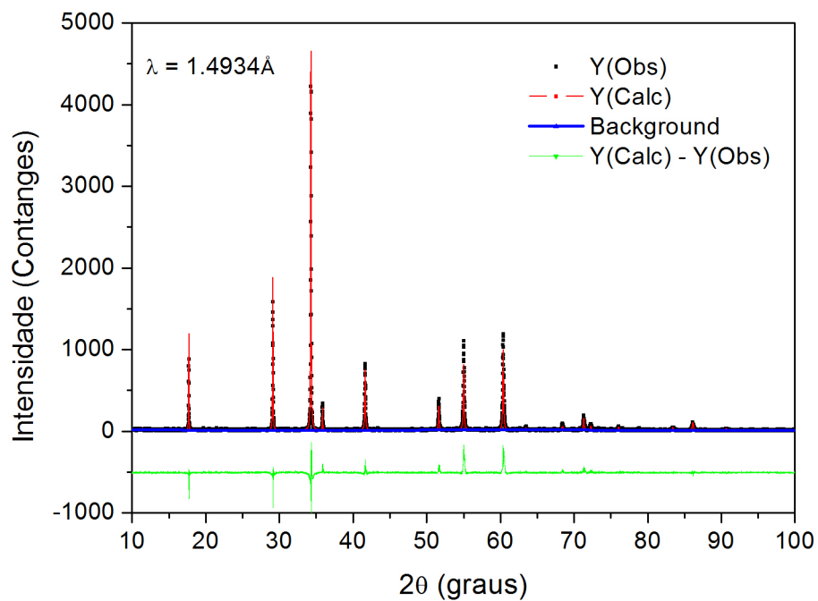
Figura 21 – Difratoograma experimental (preto), calculado (vermelho), a diferença entre o calculado e o observado (verde) e o background (azul), para a amostra NM900 analisada com radiação na borda de absorção do níquel ( 1,4934\text{\AA} ).
