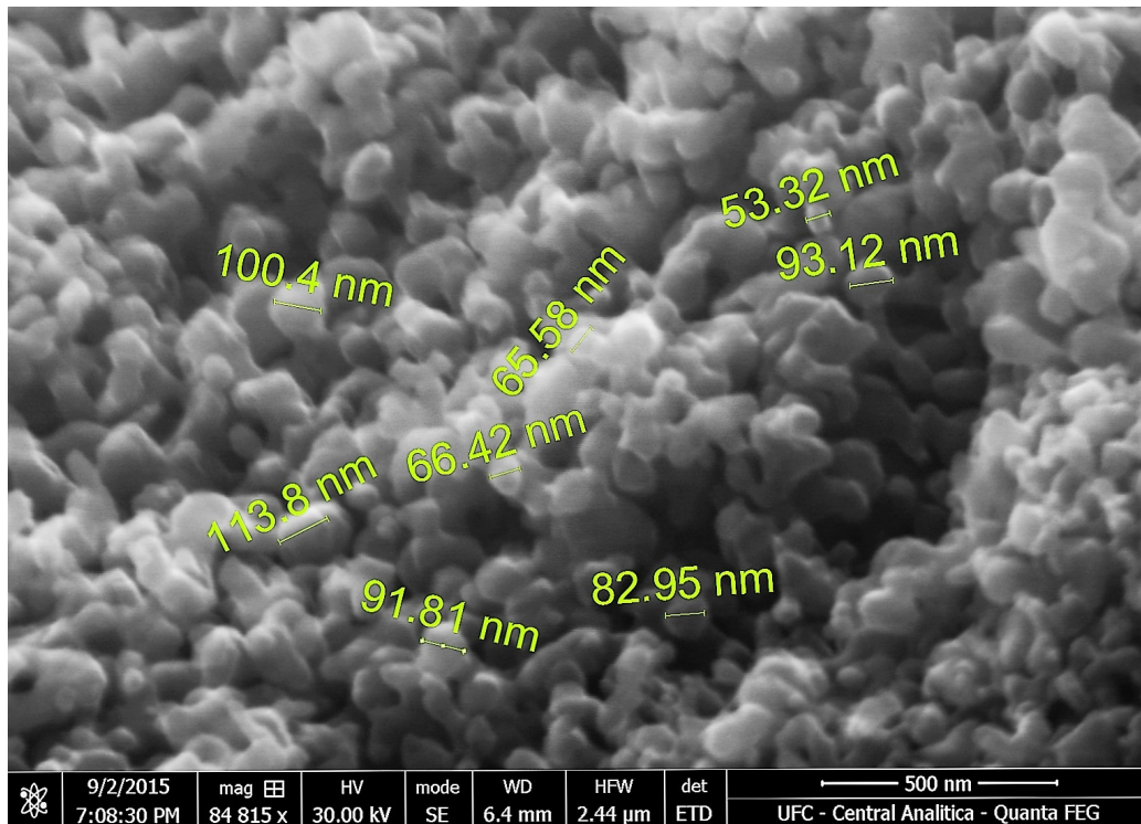
Figura 27 – Micrografia da amostra N85CM900.
