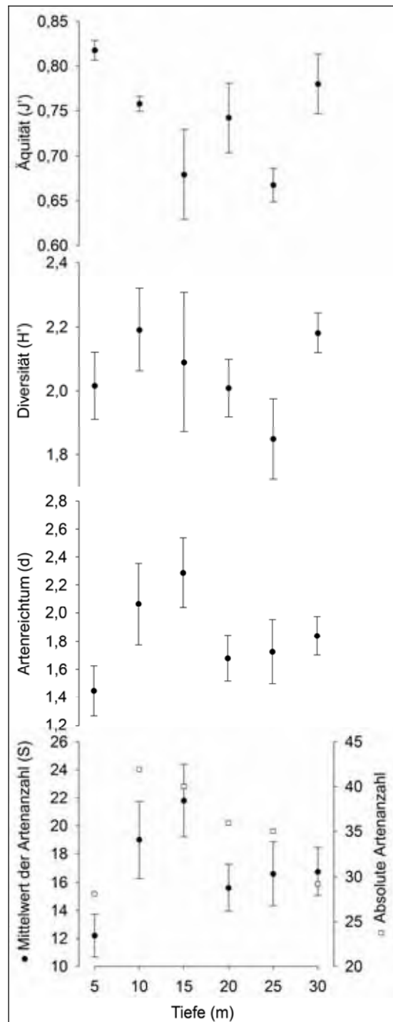
Abb. 9: Dargestellt sind die absolute Artenanzahl, der Mittelwert der Artenzahl (S), sowie der Margalef Index (d), der Shannon-Wiener Index (H') und der Pielou Index (J') der jeweiligen Stationen (Tiefe in m), als Fehler ist hier der Standardfehler (SF) angegeben.
