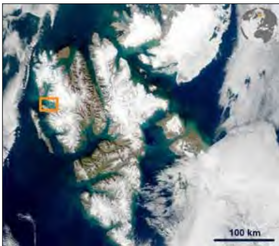
Abb. 1: Svalbard MODIS Satellitenbild, aufgenommen am 27.08.2003 aus 250 m Höhe
