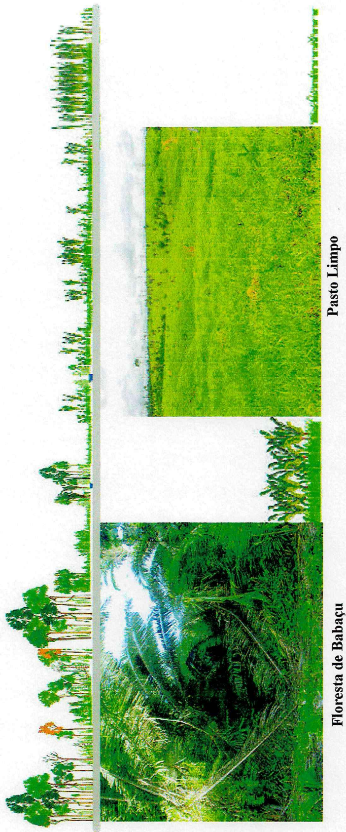
FIG. 5.3. Componentes da paisagem do PA-Benfica, Mesorregião Sudeste Paraense.
