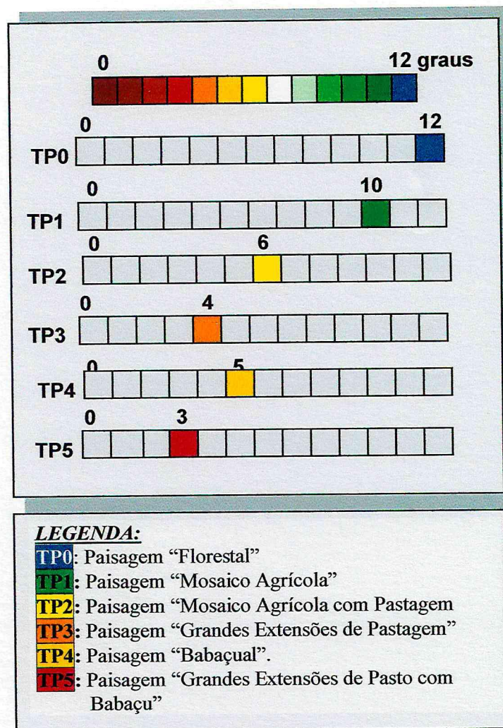
FIG. 5.14. Escala da Complexidade dos Tipos de Paisagens do PA-Benfica, Mesorregião Sudeste Paraense.
